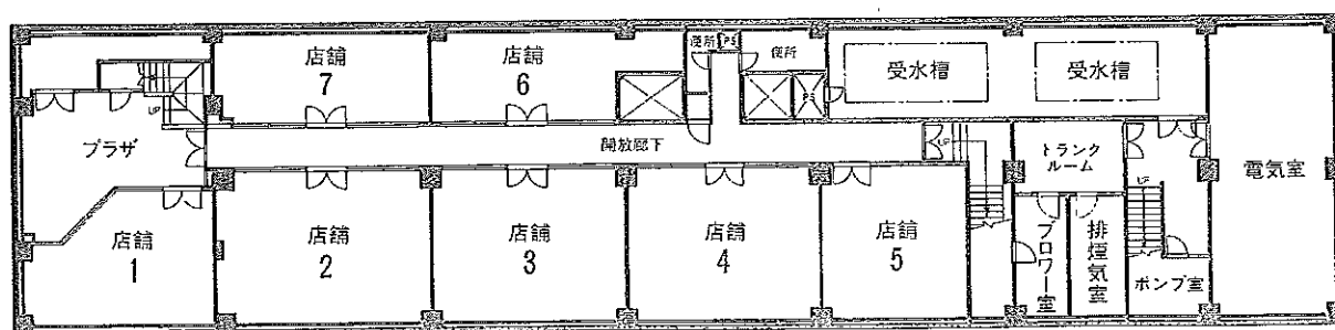
配置図・1階
